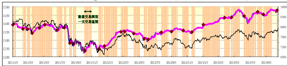
『動量交易模型』交易台灣加權股價指數累積值【20110103~20131018】
