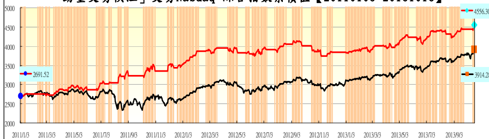
『動量交易模型』交易 Nasdaq 綜合指數累積值【20110103~20131018】
